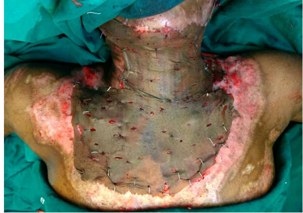
Fig. 8: Post autografting
